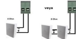
4 - 8 Ohm Terminal Bağlantı Şekilleri
