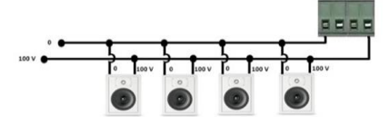
Com - 50 - 70 - 100 v Terminal Bağlantı Şekilleri
